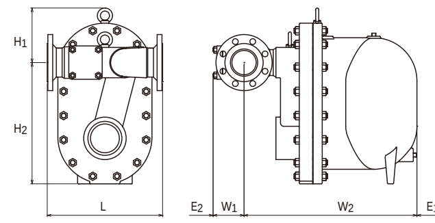
Dimensions GH70
