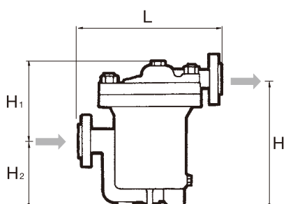
Dimensions ER25
