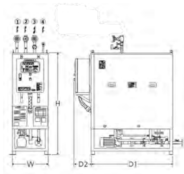
Dimensions
