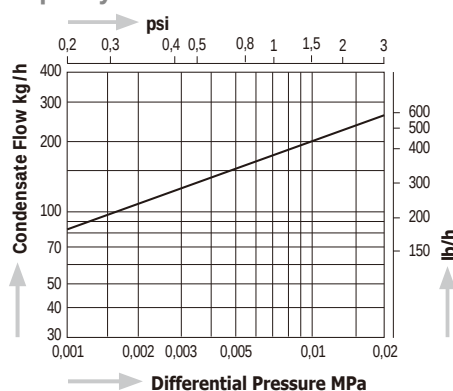
Capacity Chart F1
